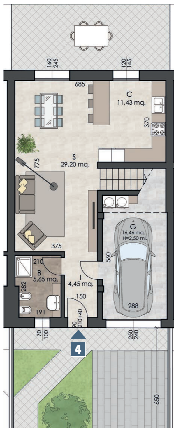
PIANO TERRA - SCALA 1:100
