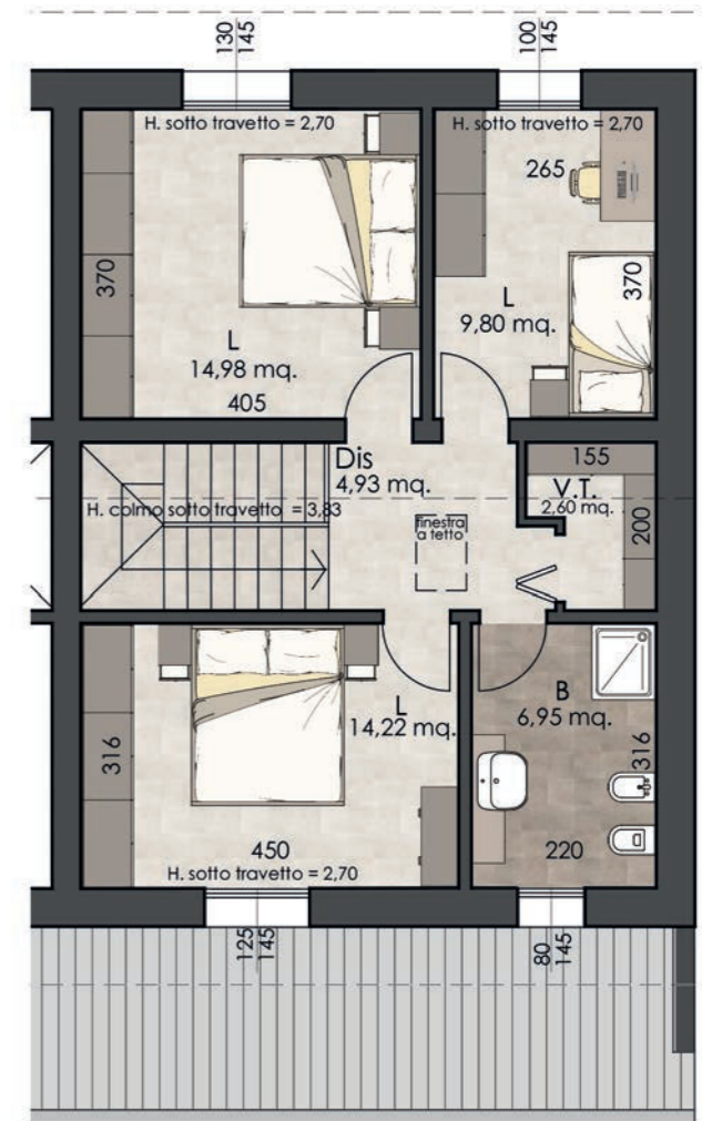
PIANO PRIMO - SCALA 1:100
